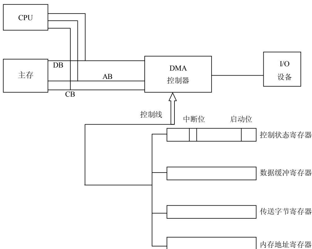
图 5.2 DMA 控制器与其他部件的关系
