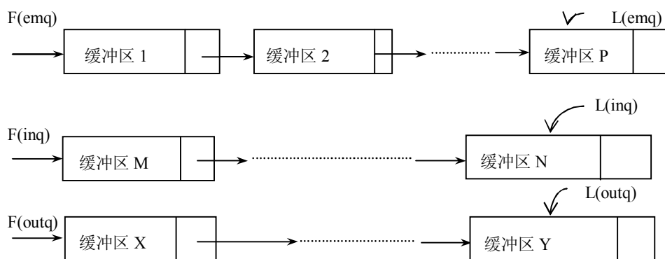
图 5.5 缓冲区队列缓冲区
