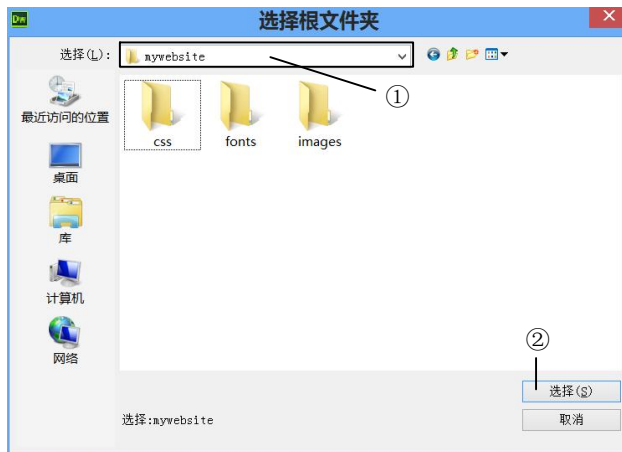
图 2-16 “选择根文件夹”对话框
