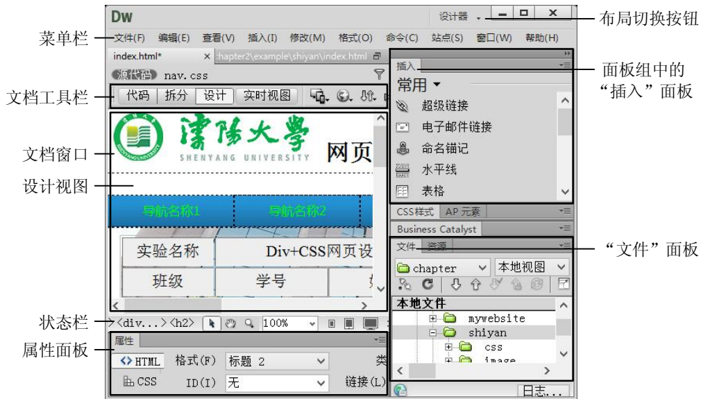
图 2-2 Dreamweaver CS6 主界面
